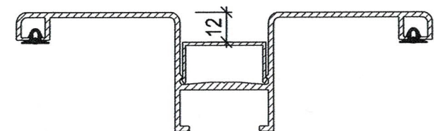
Zusammenbau Lisene 160 Artikel Nr. 14.004 + Abdeckkappe klein Artikel Nr. 14.003 + Dichtgummi Artikel Nr. 14.005
