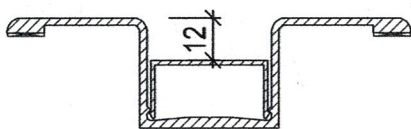
Zusammenbau Lisene 110 Artikel Nr. 14.001 + Abdeckkappe klein Artikel Nr. 14.003 + ggf. Dichtung mit Kompriband
