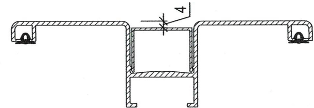
Zusammenbau Lisene 160 Artikel Nr. 14.004 + Abdeckkappe klein Artikel Nr. 14.003 + Dichtgummi Artikel Nr. 14.005
