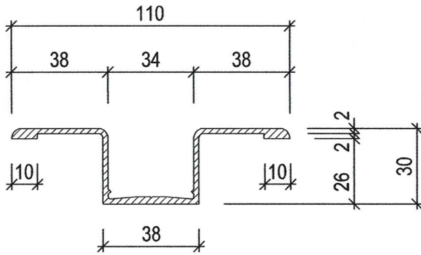
Lisene 110 Artikel Nr. 14.001
