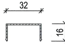
Abdeckkappe klein Artikel Nr. 14.003
