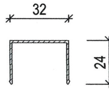
Abdeckkappe groß Artikel Nr. 14.002
