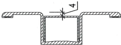
Zusammenbau Lisene 110 Artikel Nr. 14.001 + Abdeckkappe groß Artikel Nr. 14.002 + ggf. Dichtung mit Kompriband
