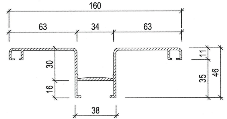
Lisene 160 Artikel Nr. 14.004
