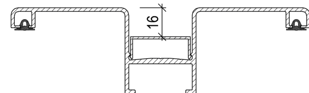
Zusammenbau Lisene 160 Artikel Nr. LIS 160 + Abdeckkappe klein Artikel Nr. LIS 116-N + Dichtgummi
