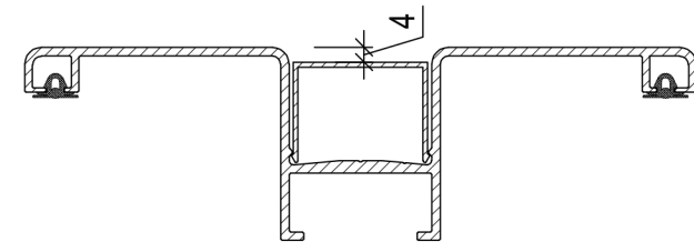
Zusammenbau Lisene 160 Artikel Nr. LIS 160 + Abdeckkappe klein Artikel Nr. LIS 116-N + Dichtgummi
