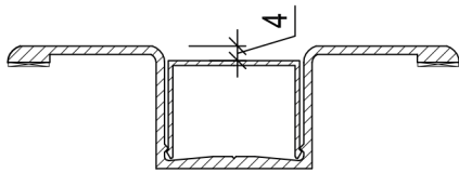
Zusammenbau Lisene 110 Artikel Nr. LIS 110 + Abdeckkappe groß Artikel Nr. LIS 110-H + ggf. Dichtung mit Kompriband
