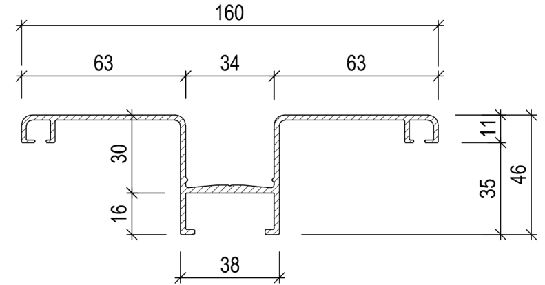
Lisene 160 Artikel Nr. LIS 160
