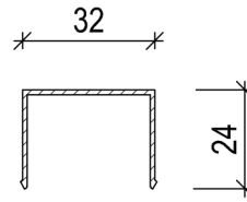
Abdeckkappe groß Artikel Nr. LIS 110-H
