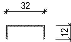
Abdeckkappe klein Artikel Nr. LIS 110-N
