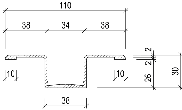
Lisene 110 Artikel Nr. LIS 110
