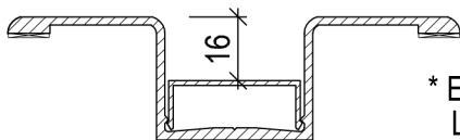
Zusammenbau Lisene 110 Artikel Nr. LIS 110 + Abdeckkappe klein Artikel Nr. LIS 110-N + ggf. Dichtung mit Kompriband*
