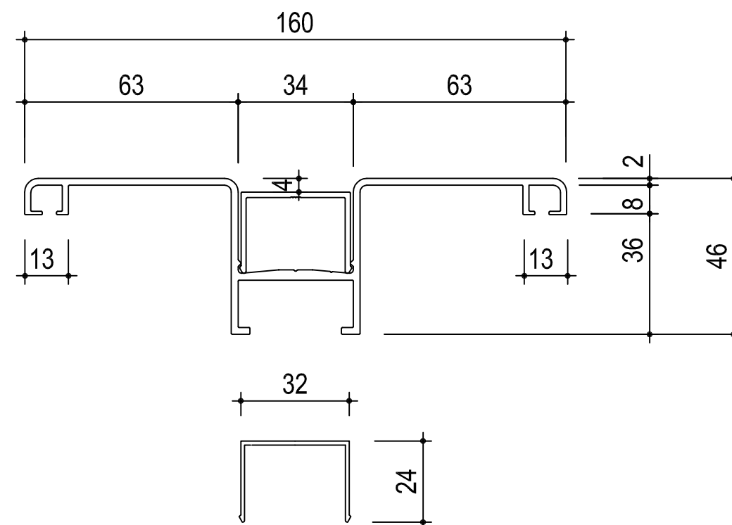
Lisene 160 + Abdeckkappe groß
