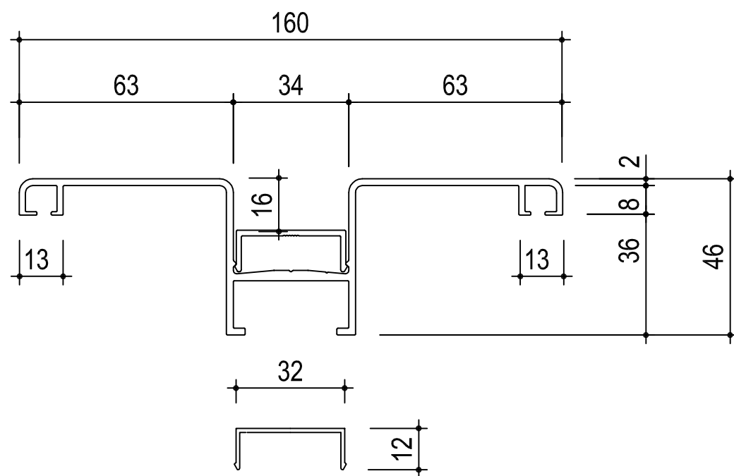
Lisene 160 + Abdeckkappe klein
