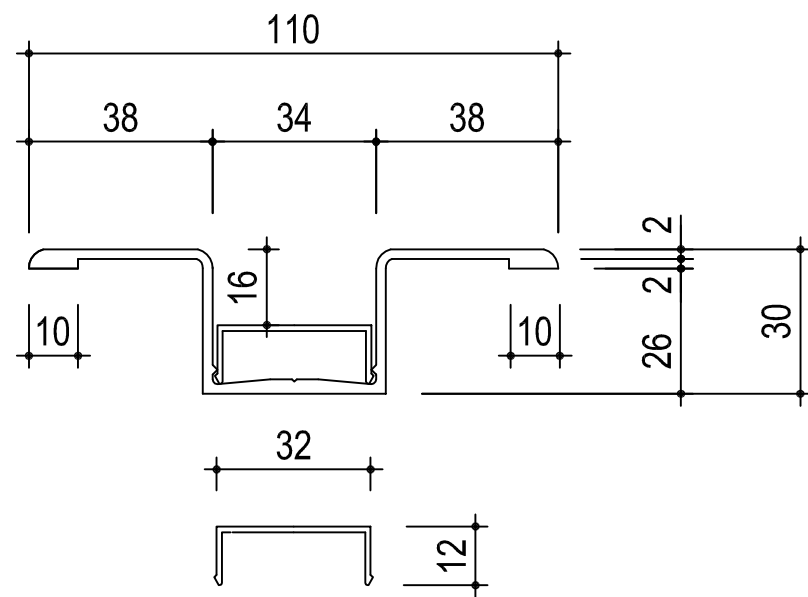
Lisene 110 + Abdeckkappe klein
