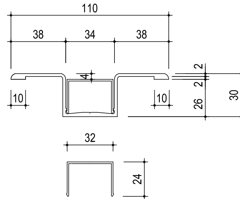
Lisene 110 + Abdeckkappe groß
