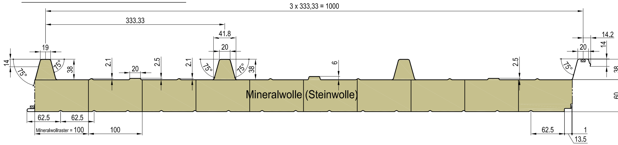
Trapezprofil A38-333
